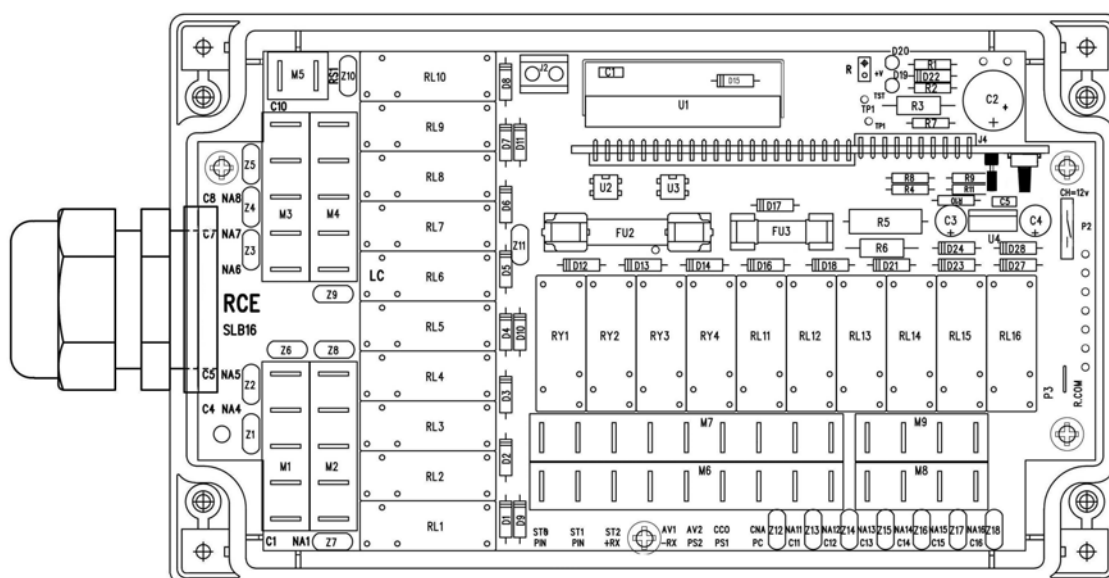
Figura 3b : Ricevitore RSL16 : vista interna
